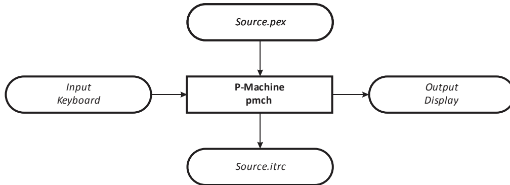
Figure 1. P-Code Interpreter
